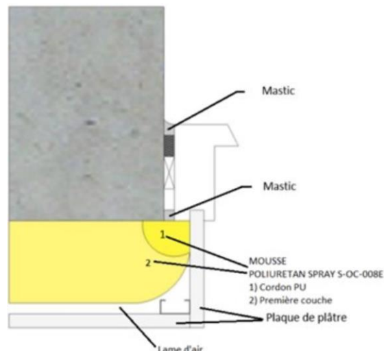
Figure 3 : Menuiserie calfeutrée en tunnel, fixée en tableau
