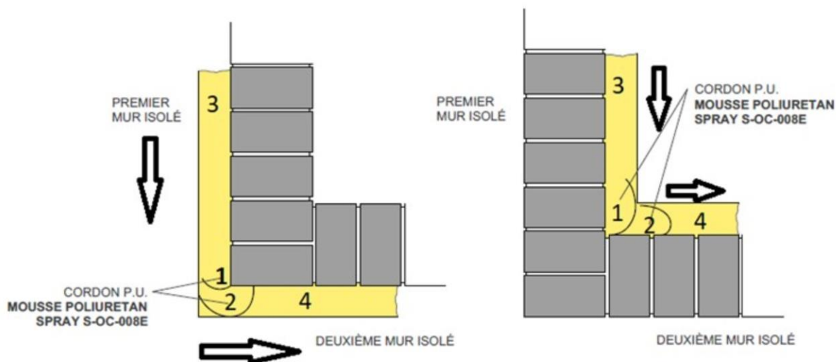
Figure 4 : Traitement des angles saillants et des angles rentrants
