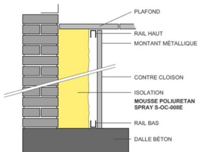
Figure 5 : Traitement de la jonction avec le plafond
