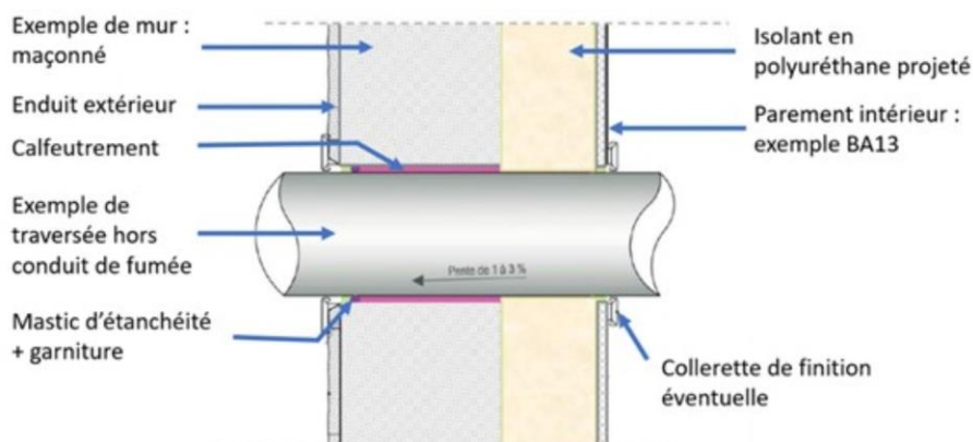
Figure 6 : Traversée de murs maçonnés : éléments autres que les conduits de fumées
