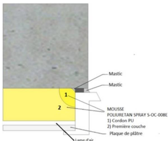
Figure 2 : Menuiserie calfeutrée en applique intérieure, fixée en applique intérieure.
